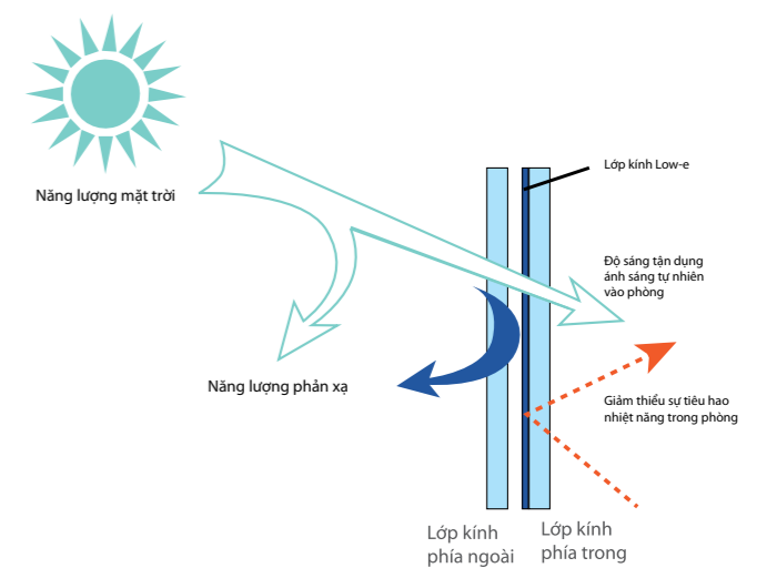
Công dụng của kính low-e nằm trong hộp kính
